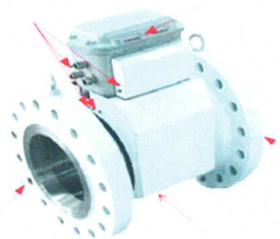
Рисунок 1 – Общий вид ПР с указанием мест пломбировки
